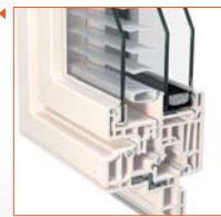
finestra accoppiata Top 72 Twin-line Classic ad elevato isolamento termoacustico e veneziana integrata, protetta dagli eventi atmosferici
